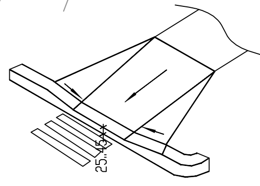
Устройство пандусов и съездов с тротуаров на проезжую часть.
