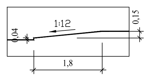
Устройство пандусов и съездов с тротуаров на проезжую часть.
